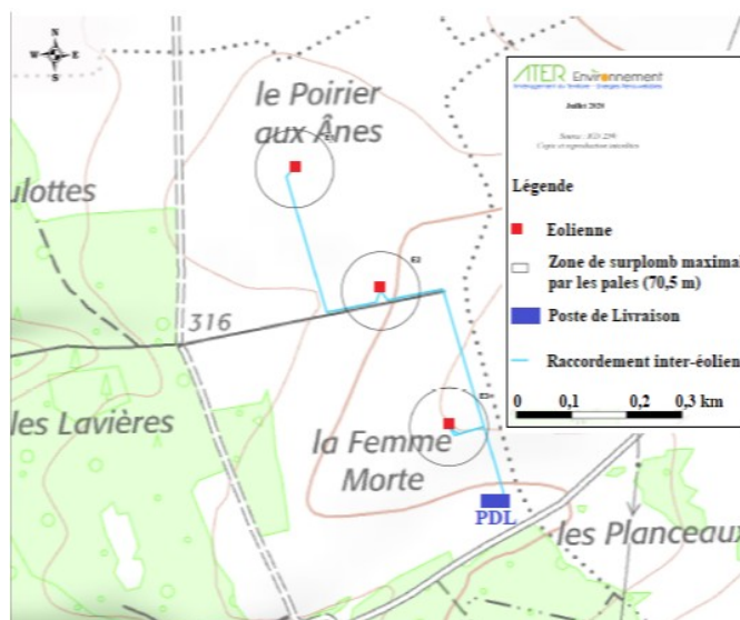
Raccordement inter-éolien (source : Etude d'impact)
