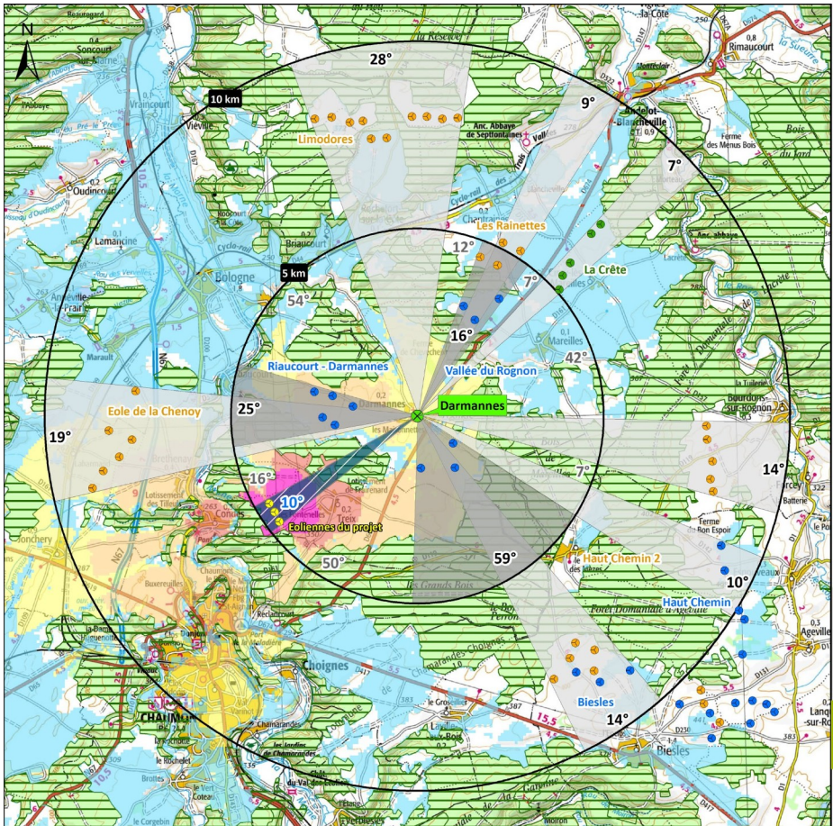
Diagramme de saturation pour la commune de Darmannes
